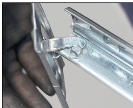
pieds en métal (hauteur 3028 mm)
